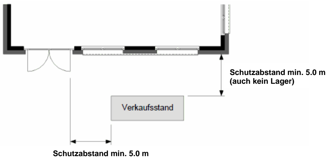
Grundriss
