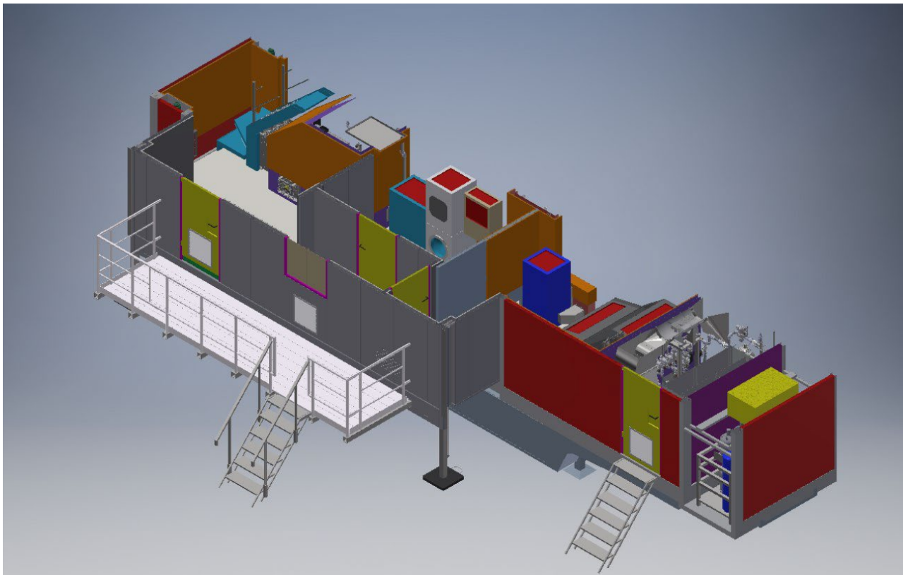
(3D-Skizze der neuen MBA; Firma Fire Go GmbH)
